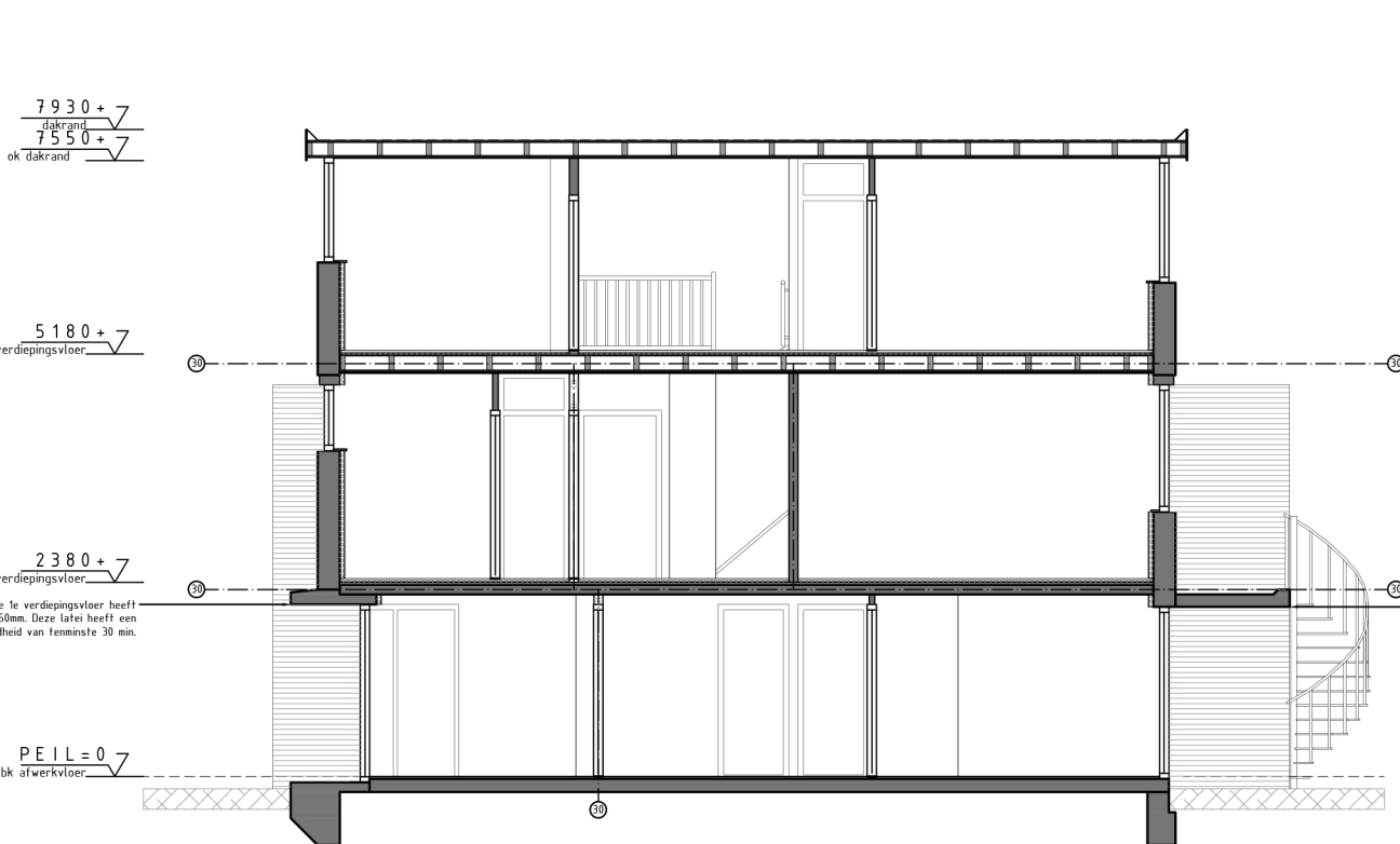
doorsnede A-A
