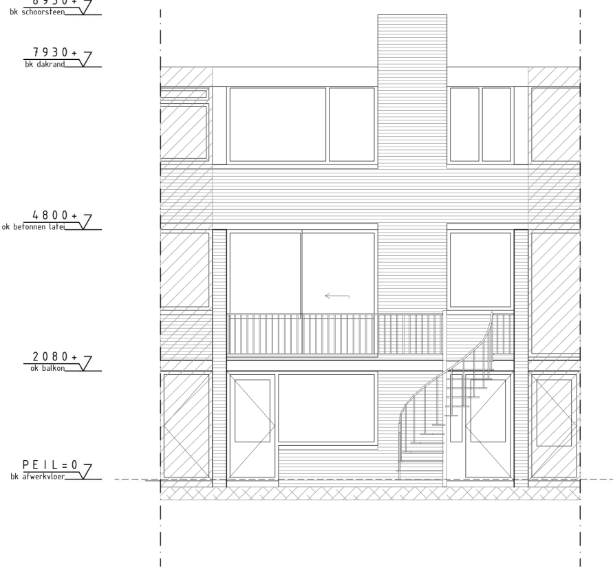
achtergevel
