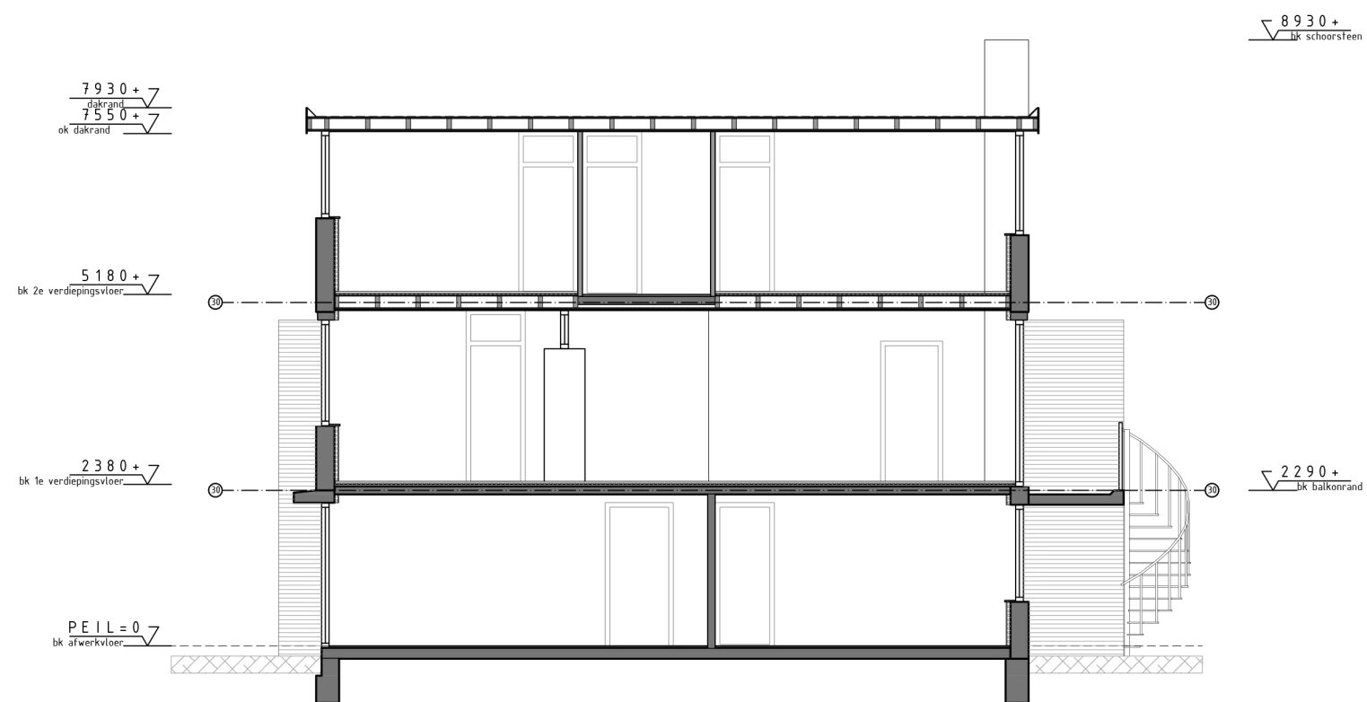
doorsnede B-B
