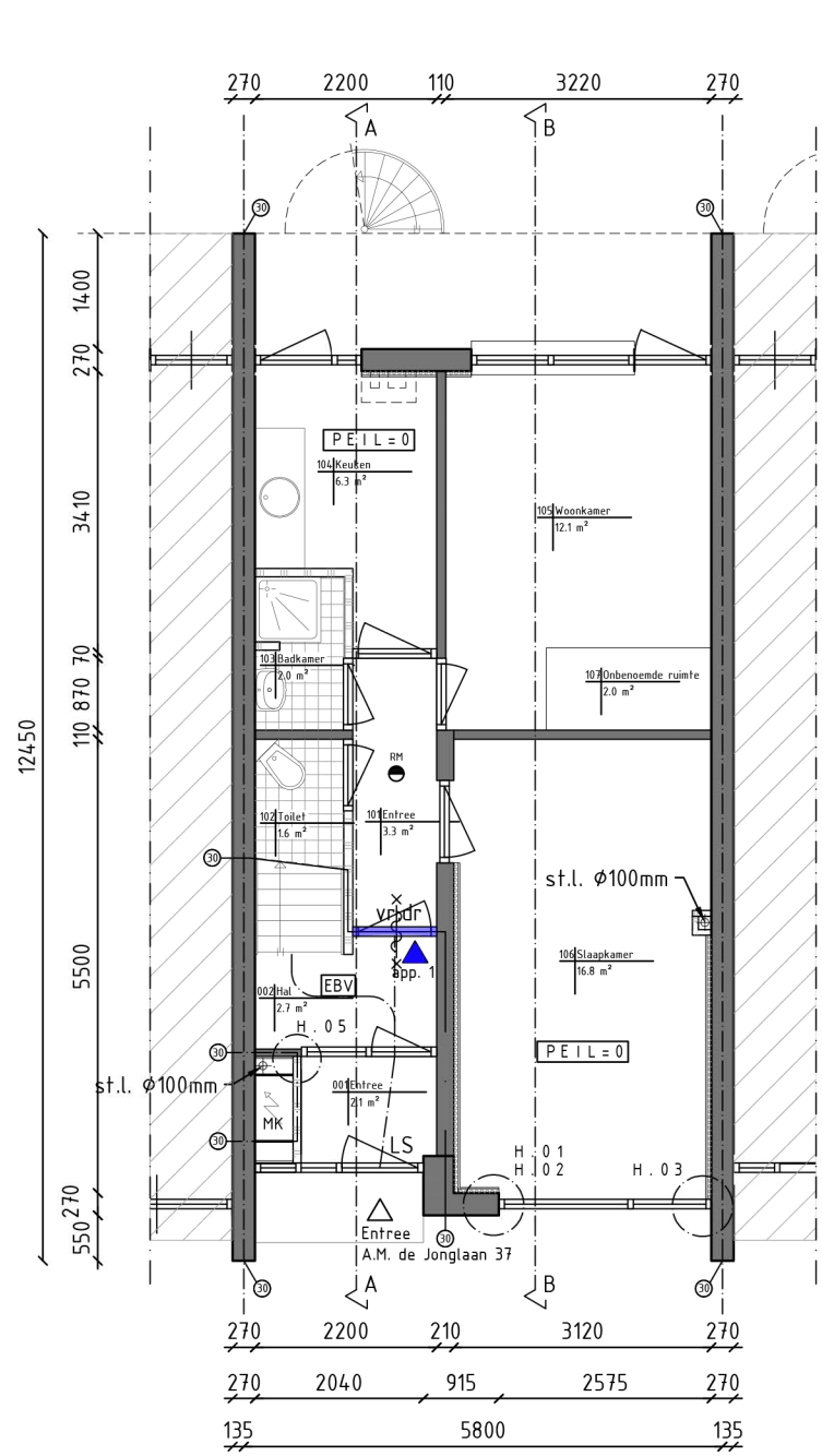
begane grond
