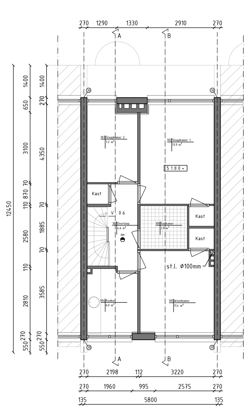
2e verdieping
