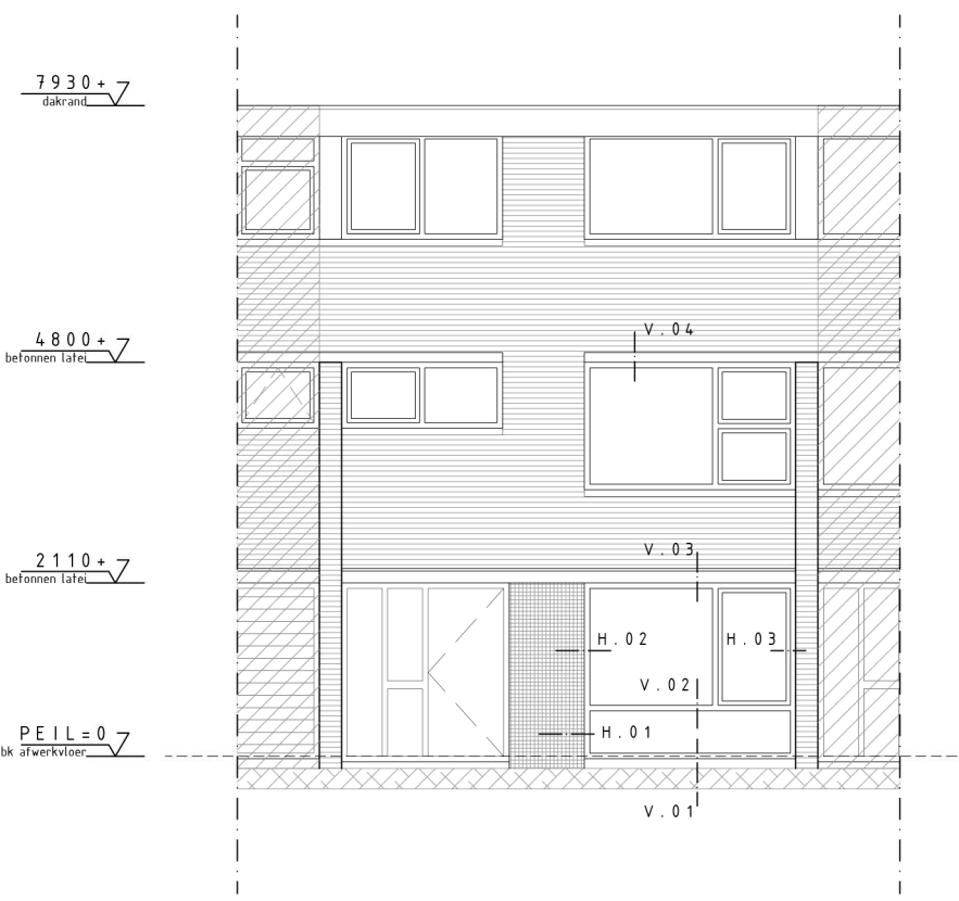
voorgevel
